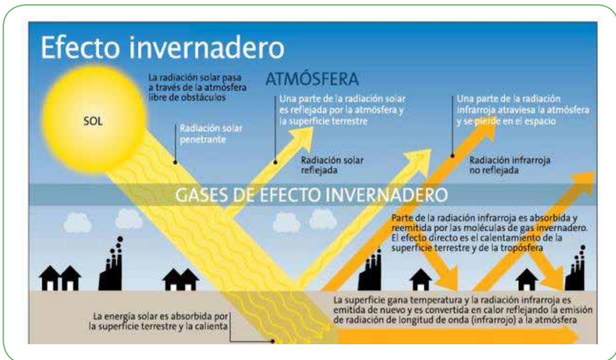
Gráfico 3: Ejemplo de funcionamiento del efecto invernadero. Fuente: UNED - GRIP - Arendal.
