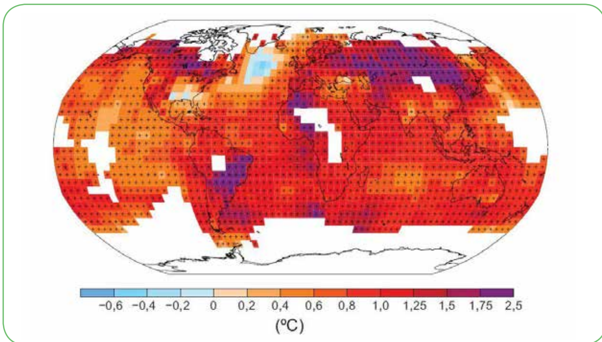
Figura 3: Variación de las temperaturas medias desde 1901 a 2012. Fuente: IPCC.
