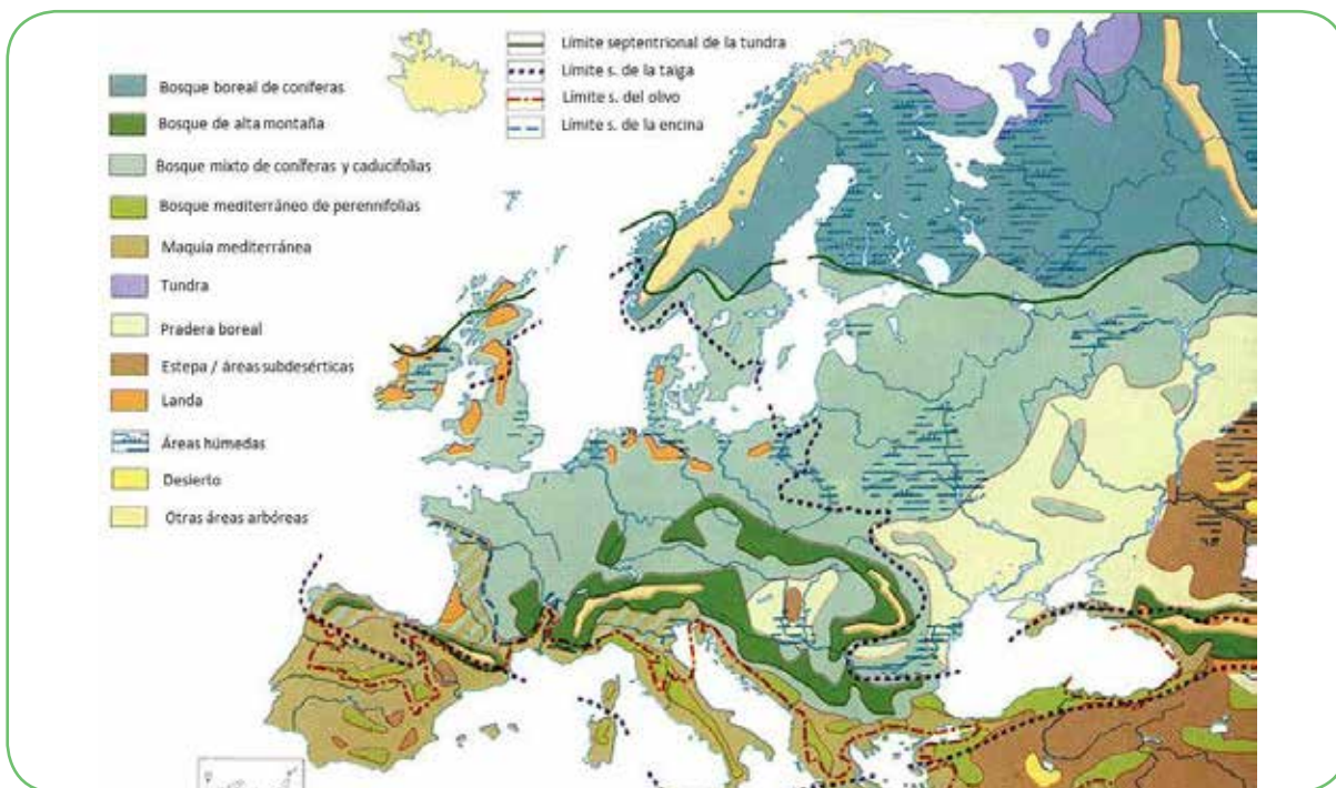
Figura 6: Mapa de las regiones biogeográficas de Europa. Fuente: Agencia Europea del Medio Ambiente.
