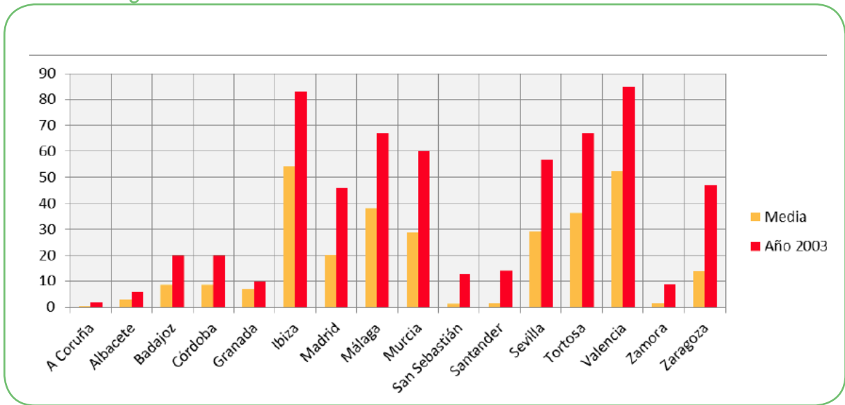
Gráfico 13: Número de noches tropicales de media para el periodo (1971 – 2000) en distintos observatorios [naranja] y número de noches tropicales en el año 2003 [rojo]. Fuente: Elaboración propia a partir de los datos de la Agencia Estatal de Meteorología.
