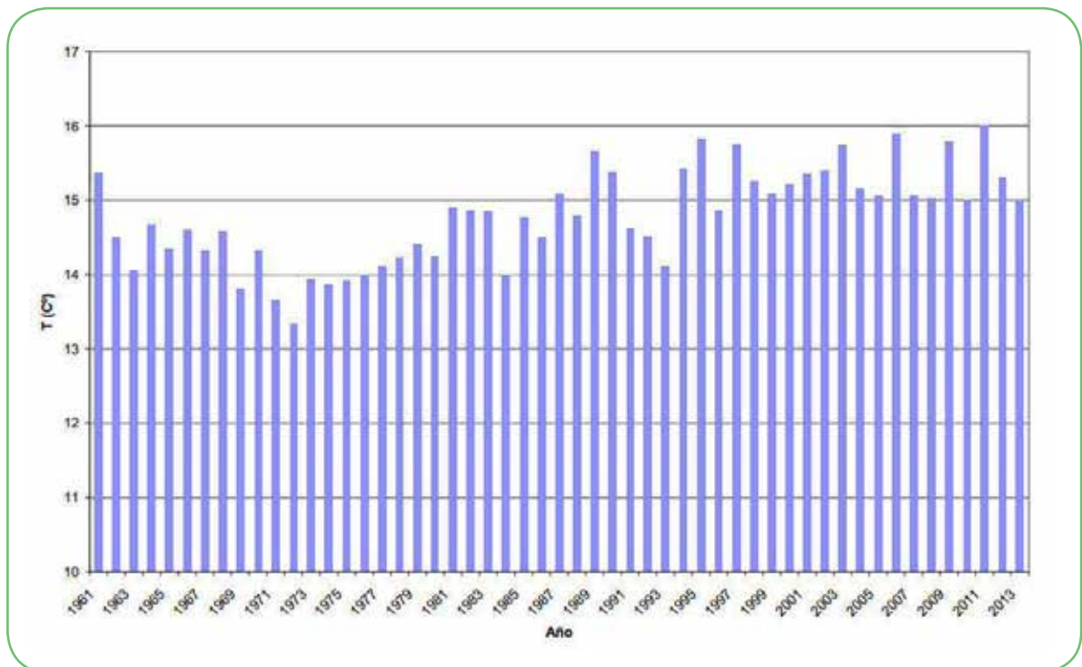
Gráfico 12: Temperatura media en España para cada año. Fuente: Agencia Estatal de Meteorología (AEMET).
