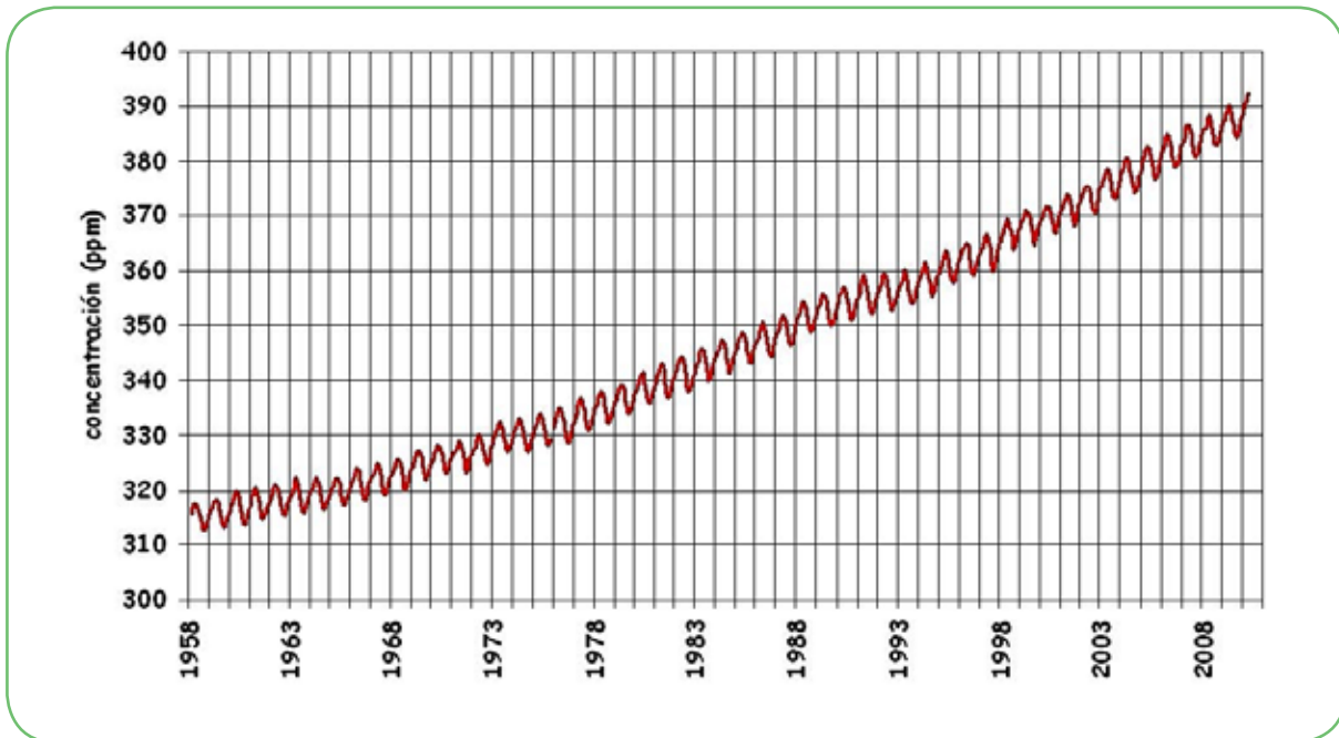
Gráfico 2: Aumento de las concentraciones de CO 2 en la atmósfera a nivel mundial desde 1958: Fuente: NOAA.
