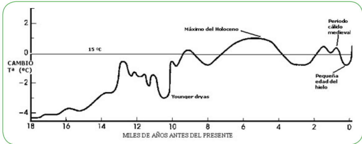
Gráfico 1: Evolución de la temperatura media del planeta en los últimos 18.000 años. Fuente: Boulton, 1993.
