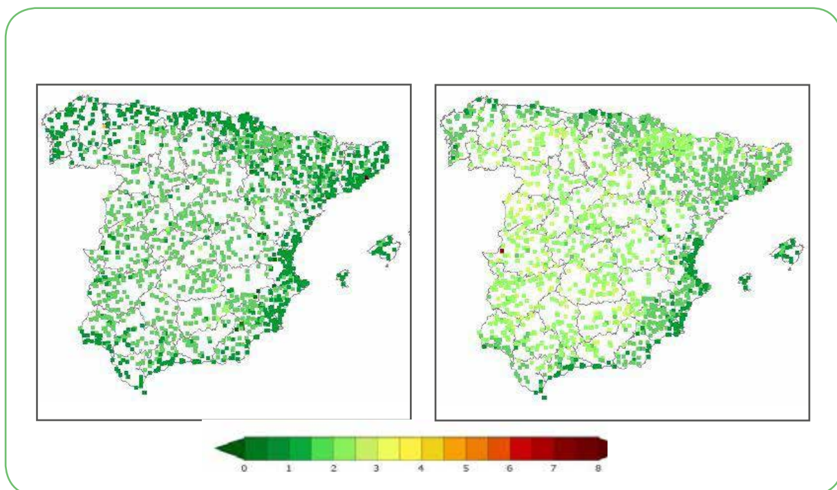
Figuras 80 y 81: Izquierda, se muestra el aumento de temperaturas previsto, de media para un escenario de bajas emisiones. Derecha se muestra también un aumento de temperaturas con emisiones altas. Fuente: Agencia Estatal de Meteorología (AEMET).
