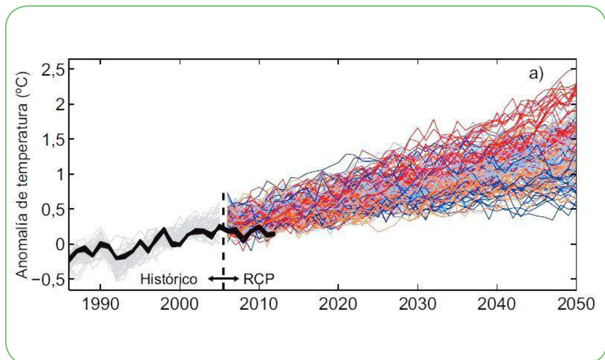
Gráfico 9: Anomalía de la temperatura desde 1980 a 2050. La línea negra es la tendencia observada. Las proyecciones se han realizado con distintos escenarios. Fuente: IPCC.
