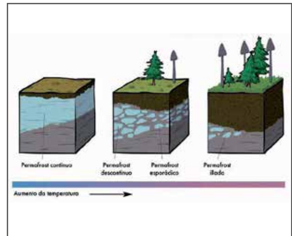
Figura 14: Secuencia de actuación del aumento de temperatura sobre el permafrost.
