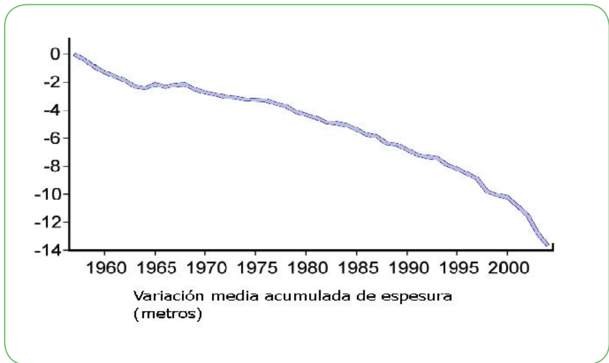
Gráfico 5: Variación media acumulada de la espesura de los glaciares (en metros) del Hemisferio Norte. Fuente: Elaboración propia.
