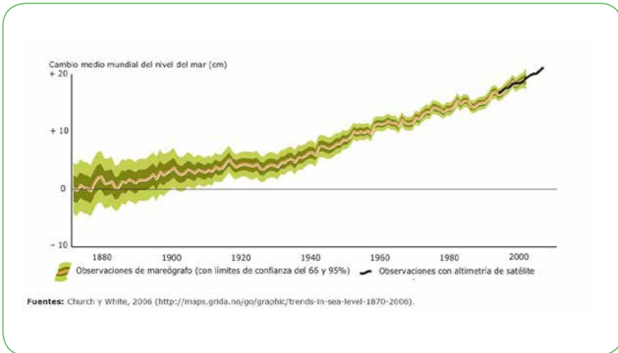
Gráfico 6: Cambios en el nivel del mar mundial 1870 – 2006. Fuente: Church y White, 2006.
