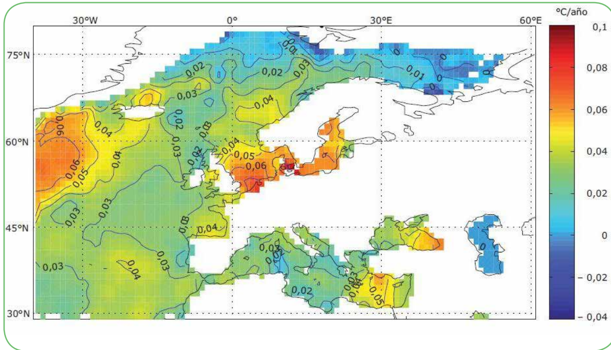
Figura 60: Aumento de las temperatura de la superficies de los mares y océanos desde que existen datos, en equivalencia de grados centígrados por año. Fuente: Coppini y Pinardi, 2007.
