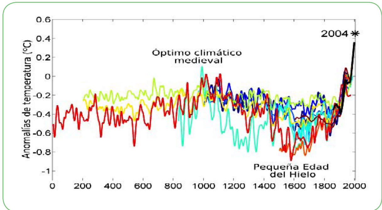
Gráfico 4: Anomalías de temperaturas sobre la superficie terrestre europea en los últimos 2000 años (diferentes modelos numéricos). Fuente: globalwarmingart
